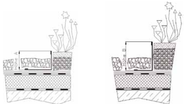
Einbauhöhe A
