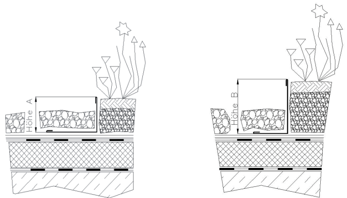
Einbauhöhe A
